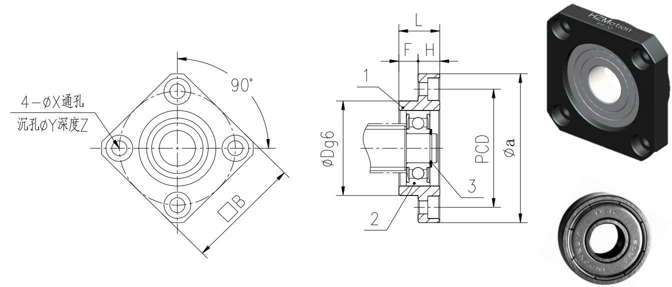
FF 型轴承座及丝杠轴端设计
